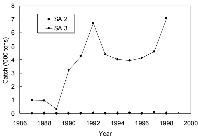
Fig. 15.1. Roughhead grenadier in Subareas 2+3: catches in Subarea 2 and Div. 3LMN.
